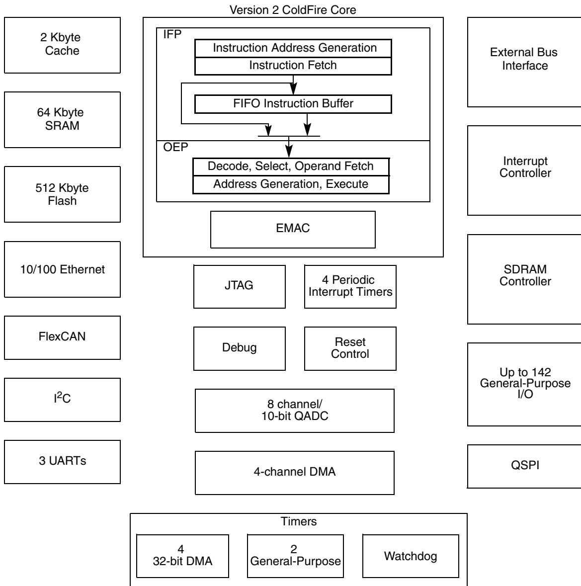
Figure 1. MCF5282 Block Diagram
